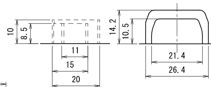
側面ロック B 詳細 (1/1)
